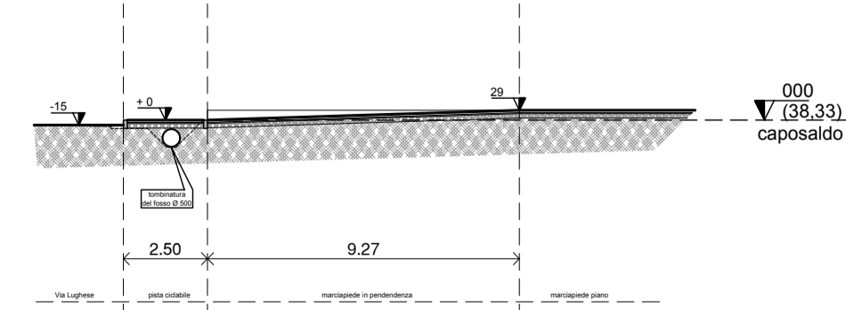
SEZIONE scala 1: 200
